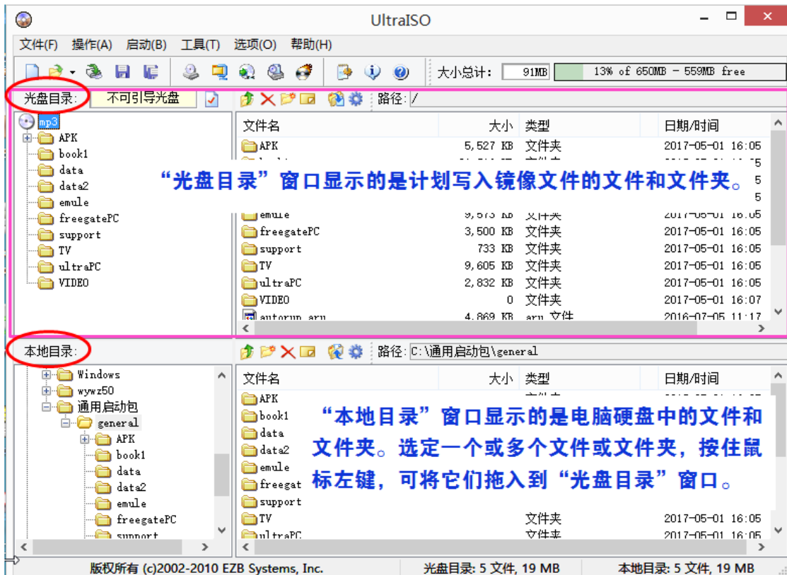
图 3-2 软件界面介绍
